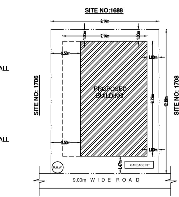
SITE PLAN (1:200)
